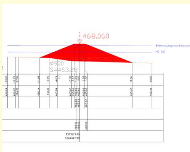
Musterquerschnitt Neuer Deich
